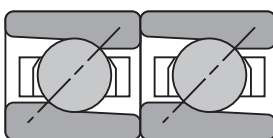
Tandem DT
