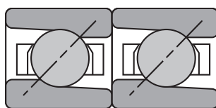
Tandem DT
