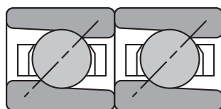
Tandem DT
