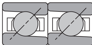
Tandem DT
