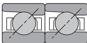
Tandem DT
