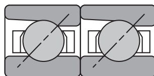
Tandem DT
