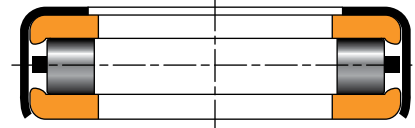
Fig. 15. Type TTSPS.
