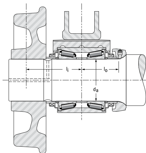
Inboard Journal
